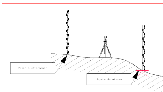
2 - Principe général du nivellement direct
