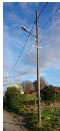
Réseau aérien BT à conducteurs isolés sur poteau bois
